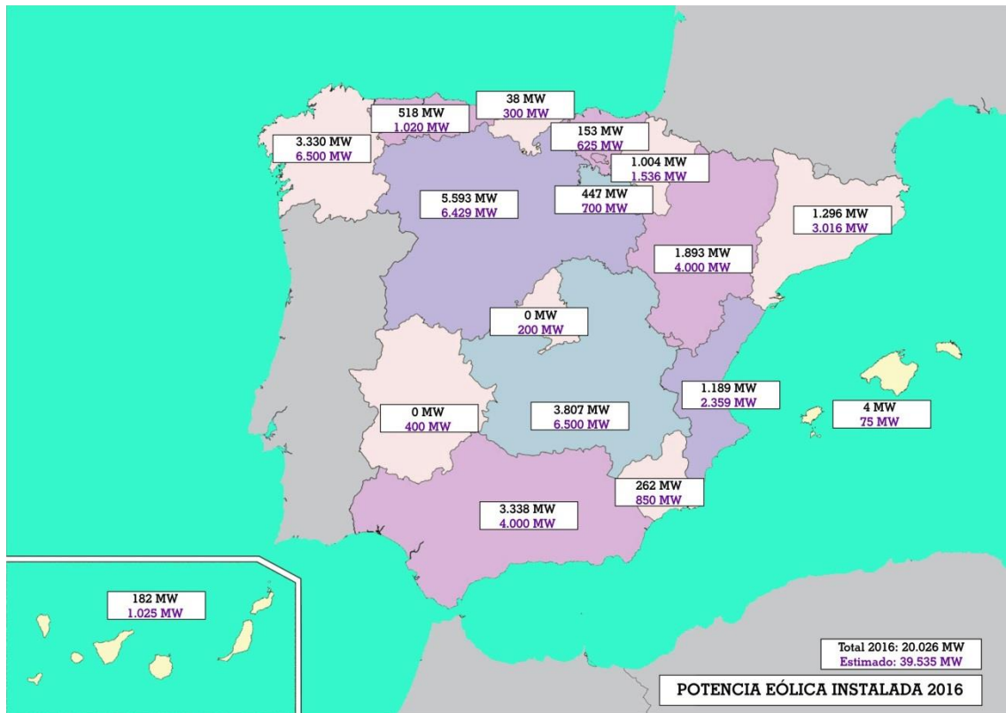
Figura 3.2.5. CCAA. Distribución de potencia eólica instalada a finales 2016 y potencial estimado.
