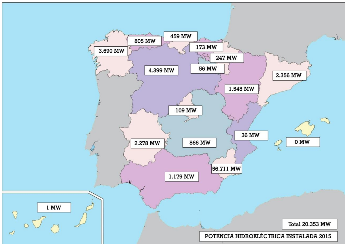
Figura 3.2.4.CCAA. Distribución de la potencia hidroeléctrica instalada a finales 2015
