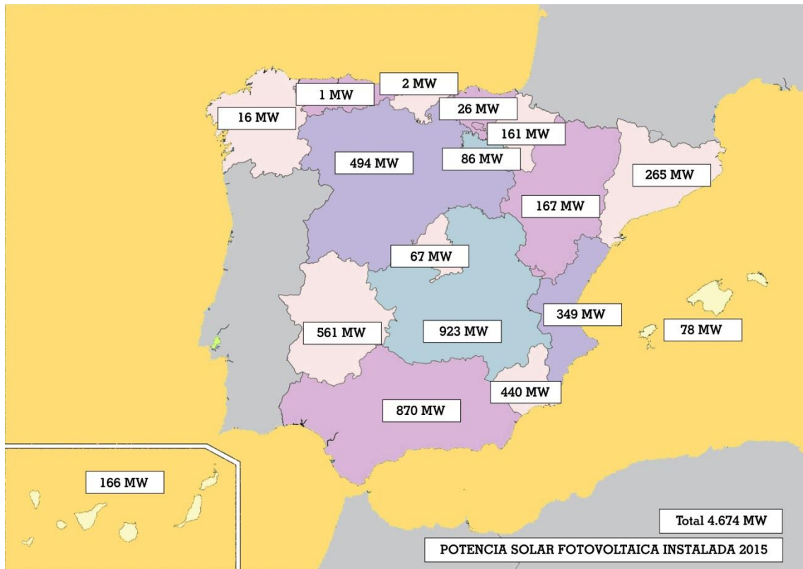
Figura 3.2.7. CCAA. Distribución de la potencia solar fotovoltaica instalada a finales 2015.
