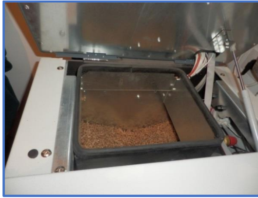
Pelletización para caldera doméstica
