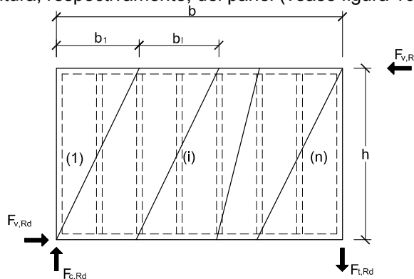
Figura 10.8 Muro diafragma
