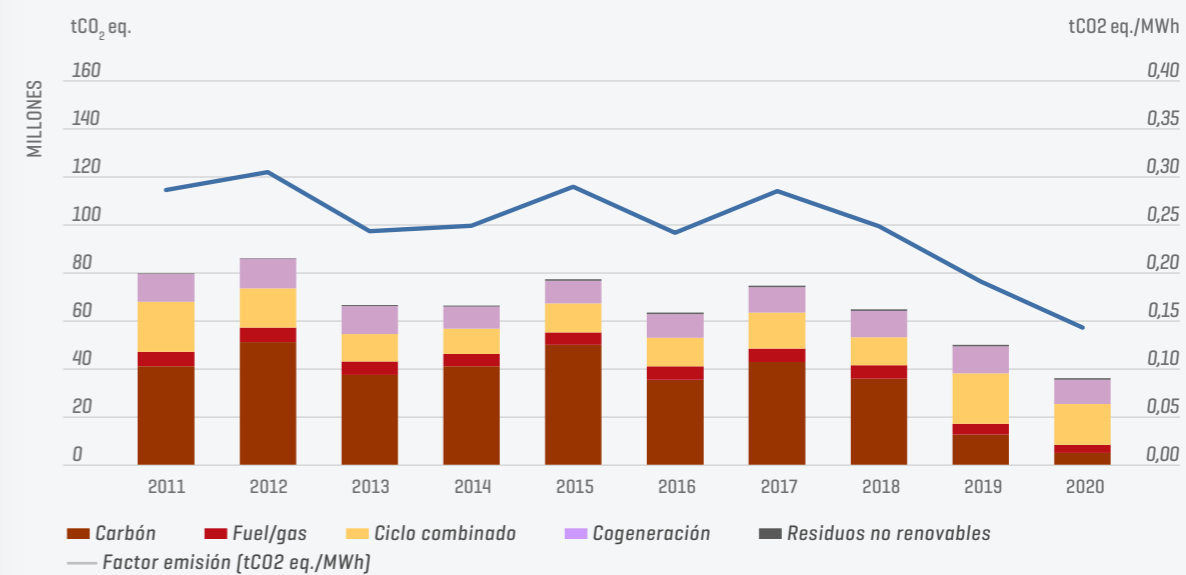
Emisiones y factor de emisión de CO 2 eq. asociado a la generación de energía eléctrica nacional [1]
